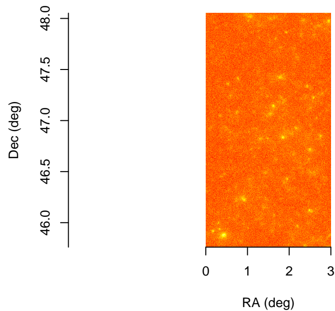
Noisy Data (sigma=10%)
