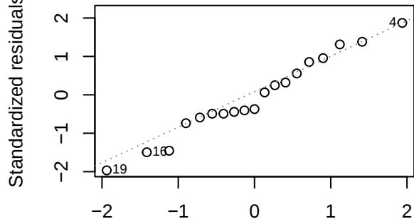
Normal Q-Q
