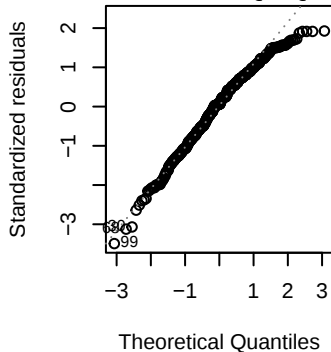
Normal Q-Q
