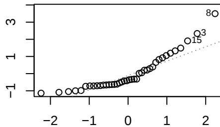
Normal Q-Q
