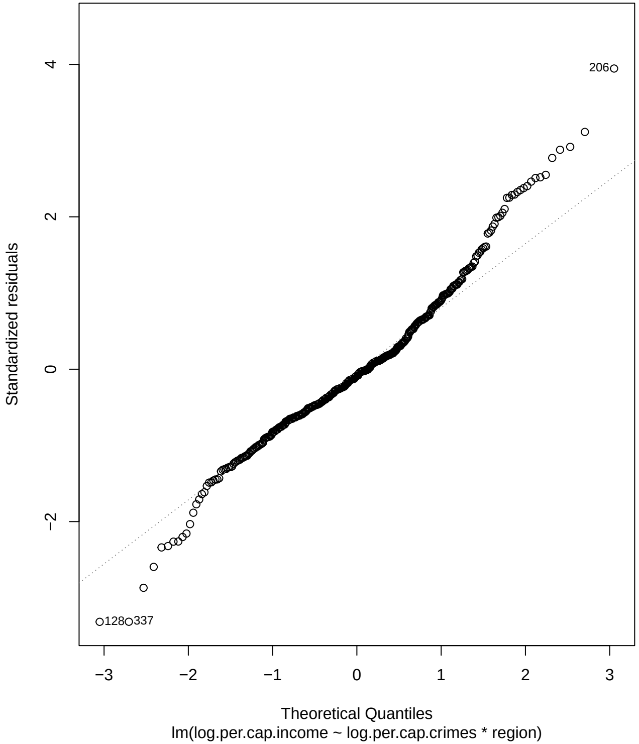
Normal Q-Q
