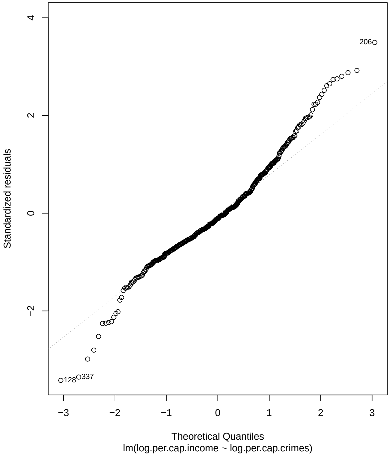
Normal Q-Q
