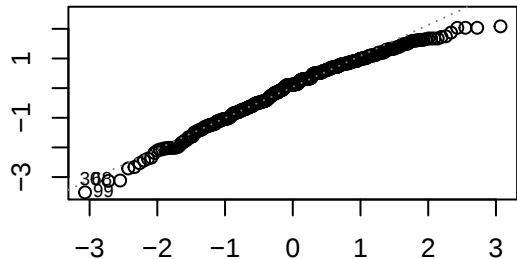
Normal Q-Q
