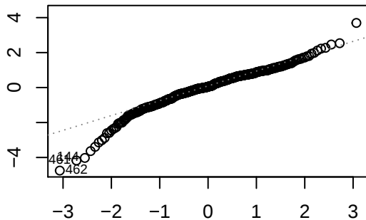
Normal Q-Q
