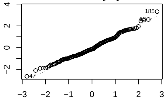
Normal Q-Q
